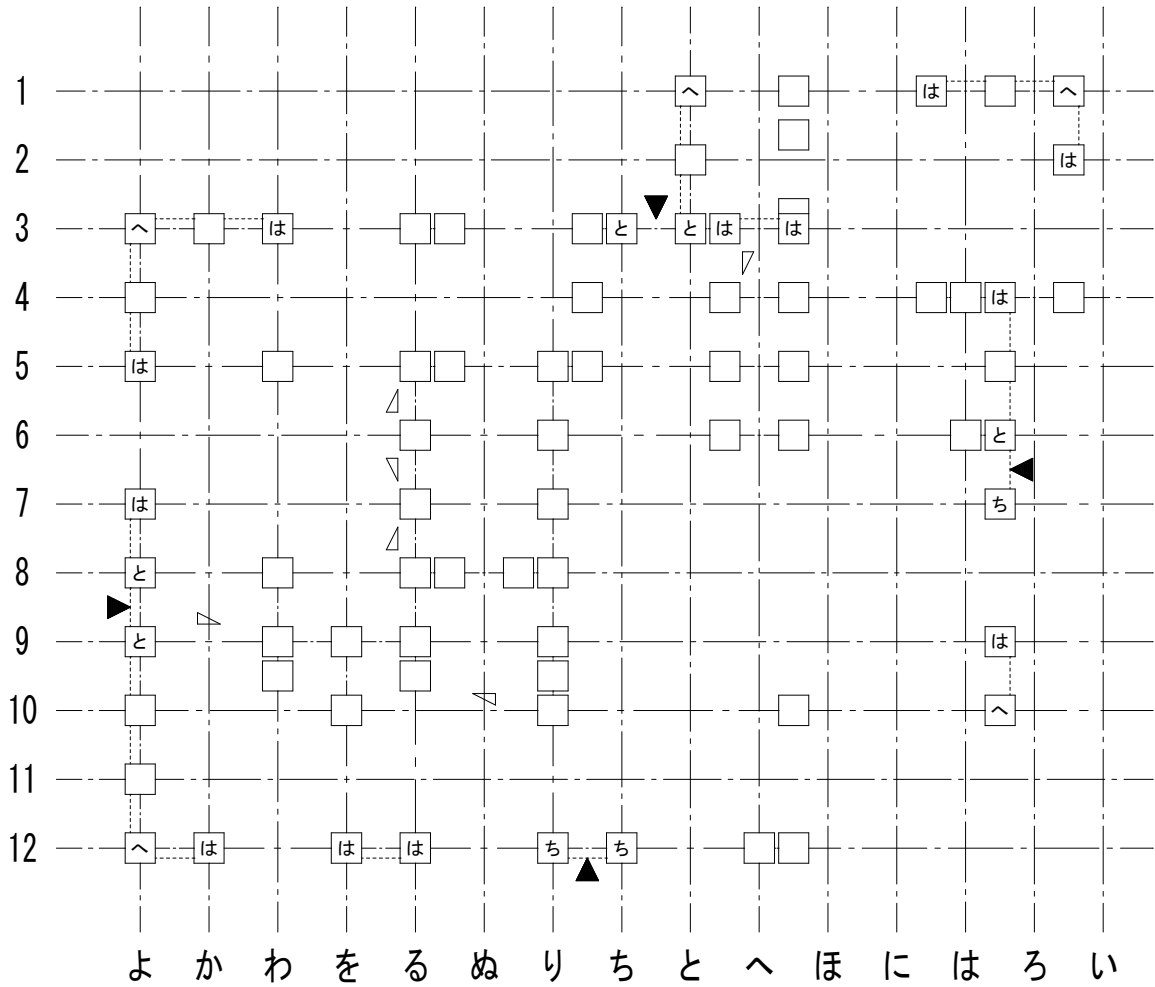
1 階柱壁伏図
